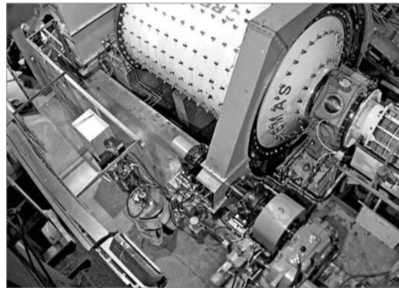
Стержневая мельница
